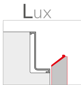
* ANTA CON PROFILO INCLINATO (OPZ. P+I+ COD. COLORE) DOOR WITH INCLINED PROFILE
